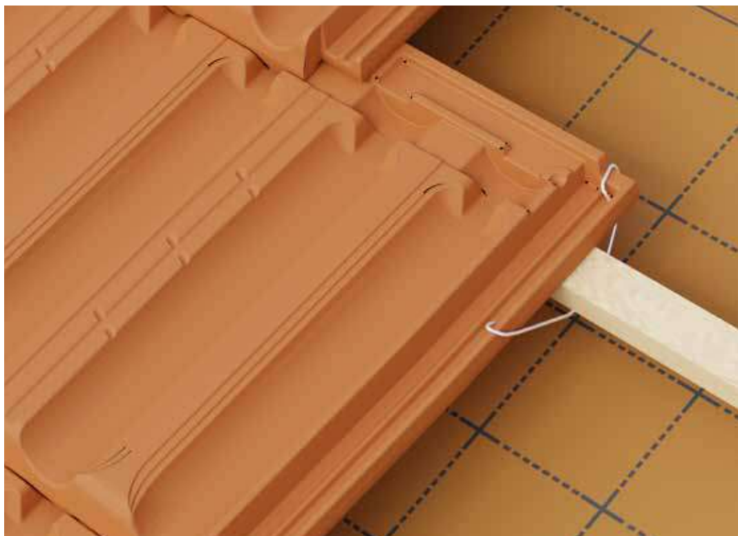
Gancio controvento per tegola in cotto sagomato
